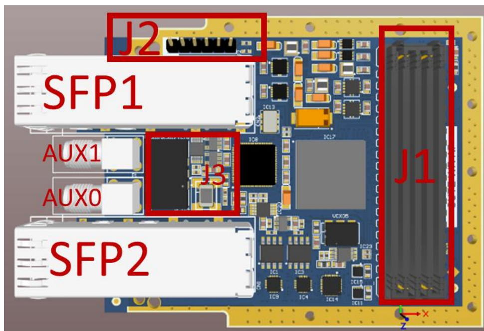
硬件接口 (CUTE-WR-A7 正面向上)
